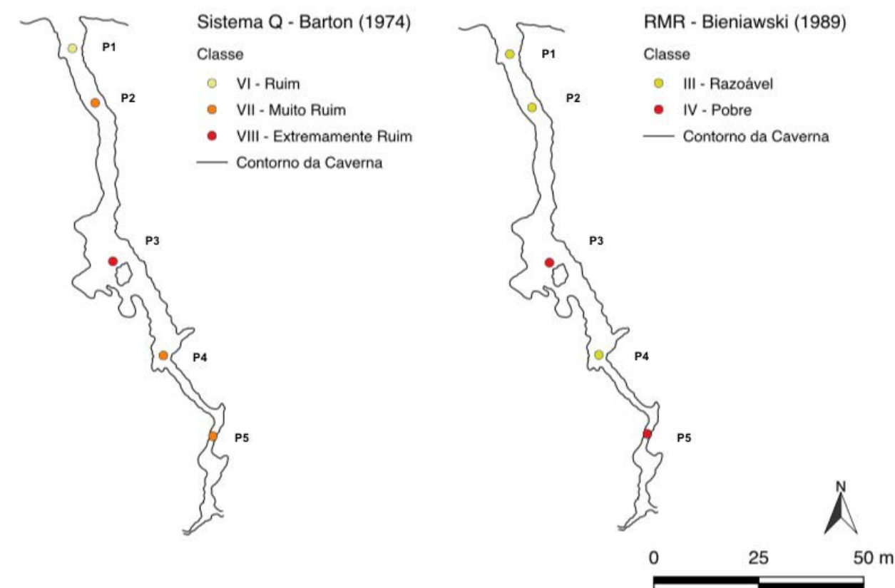
Figura 7: Classificação geomecânica Q e RMR segundo os pontos de amostragem na Gruta do Pião.
