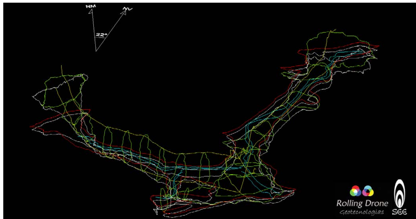
Figura 4: Perspectiva isométrica da cavidade com destaque para os vetores extraídos automaticamente no 3DReshaper.
