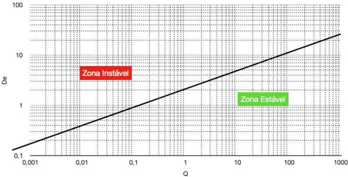
Figura 3: Gráfico de zoneamento de estabilidade que correlaciona o Diâmetro Equivalente (De) e o índice Q. Modificado de Barton et al. (1974).
