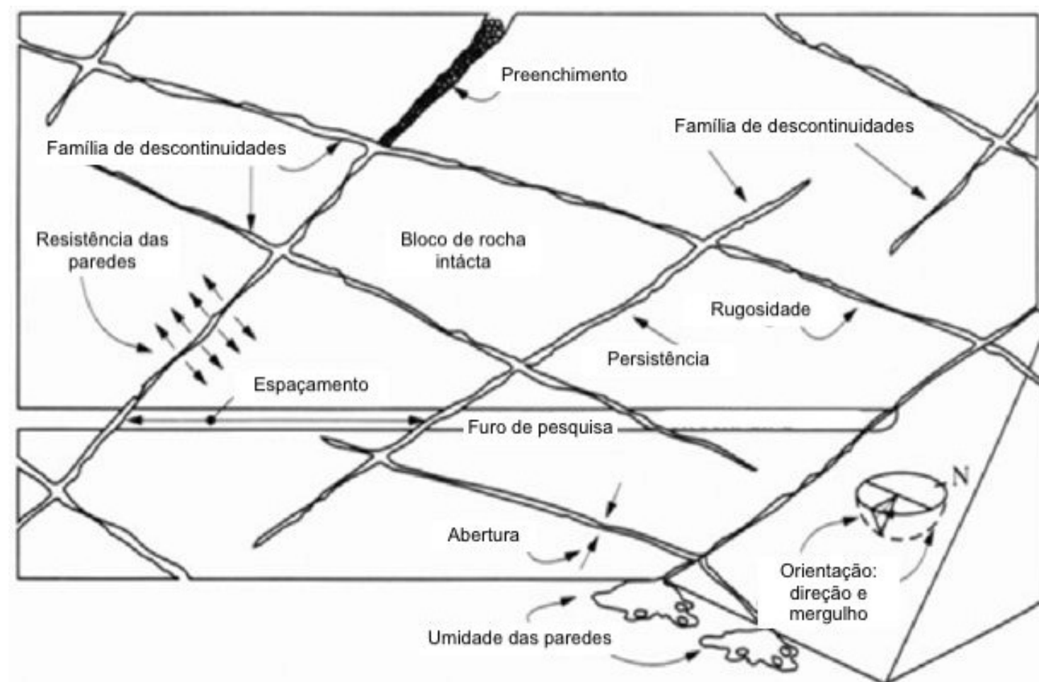
Figura 2: Bloco diagrama apresenta os principais parâmetros geomecânicos avaliados na caracterização do maciço rochoso. Modificado de Hudson (1989).
