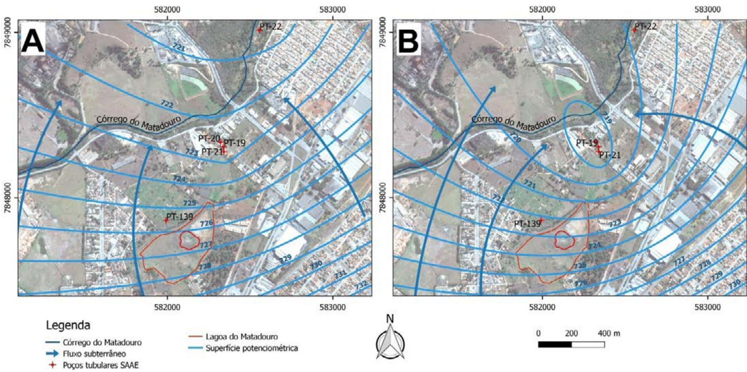
Figura 5 - Mapas da superfície potencimétrica da área de estudo indicando o sentido do fluxo da água subterrânea para N. (A) Mapa considerando os níveis estáticos (B) e mapa considerando o bombeamento do poço PT-19 após 48 horas. Fonte: Google Earth.
