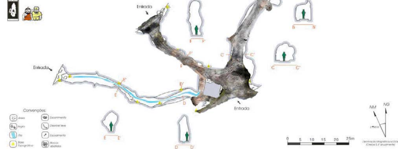
Figura 5: Sobreposição do mosaico de ortofotos do piso da Gruta dos Fugitivos sobre o mapa elaborado pelo GPME/GBPE (Modificado de Silva, 2004).
