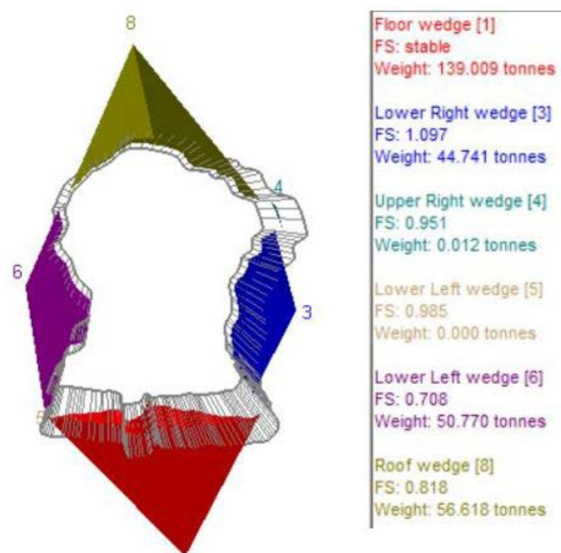
Figura 9: Análise cinemática para as cunhas formadas a partir das famílias de descontinuidades F1, F2 e F4 em P3. Os baixos valores de FS das cunhas em azul, amarelo e roxo indicam uma fragilidade geotécnica acentuada.
