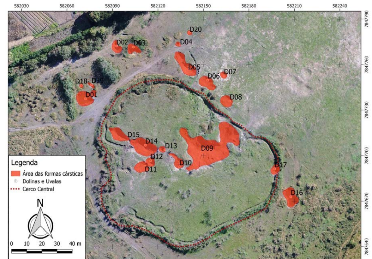
Figura 2 - Mapa das formas cársticas de recarga no interior da lagoa do Matadouro identificadas pelo sensoriamento remoto e mapeamento de campo. Fonte: Imagens obtidas por drone.
