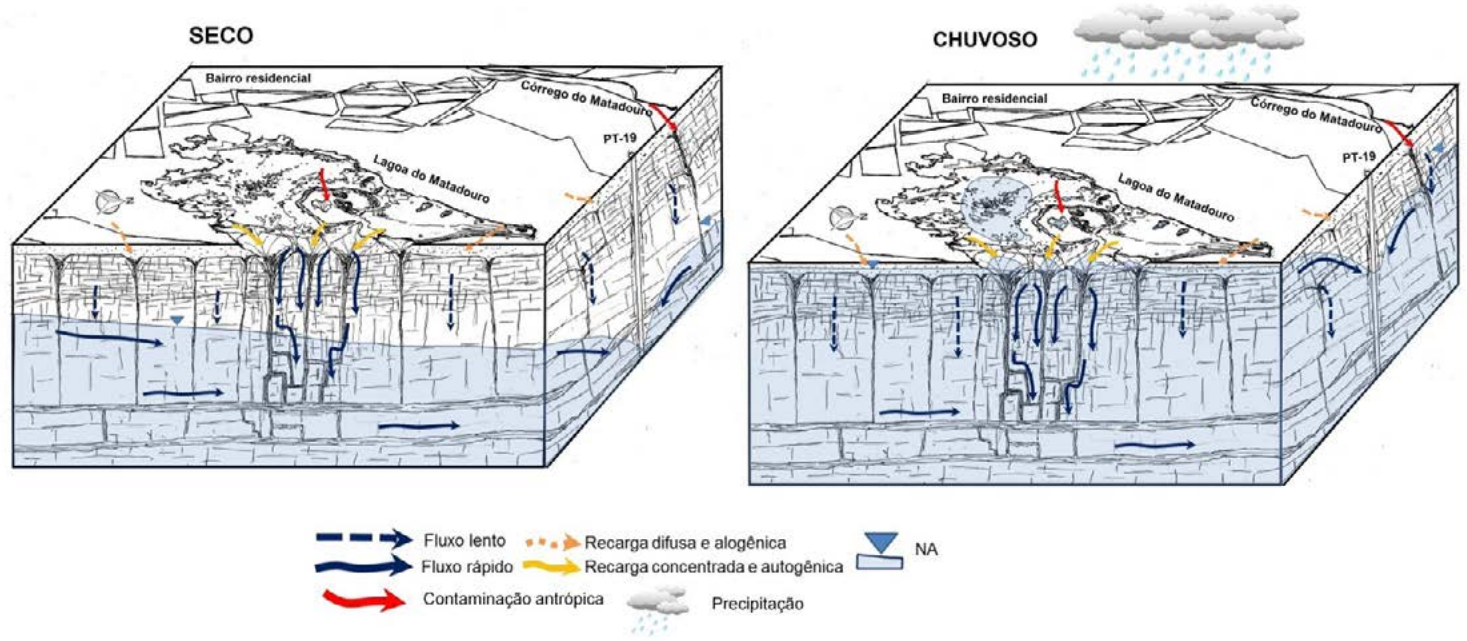
Figura 6 - Ilustração do modelo hidrogeológico conceitual da área de estudo representando todos os processos envolvidos na dinâmica hídrica do aquífero cárstico local.
