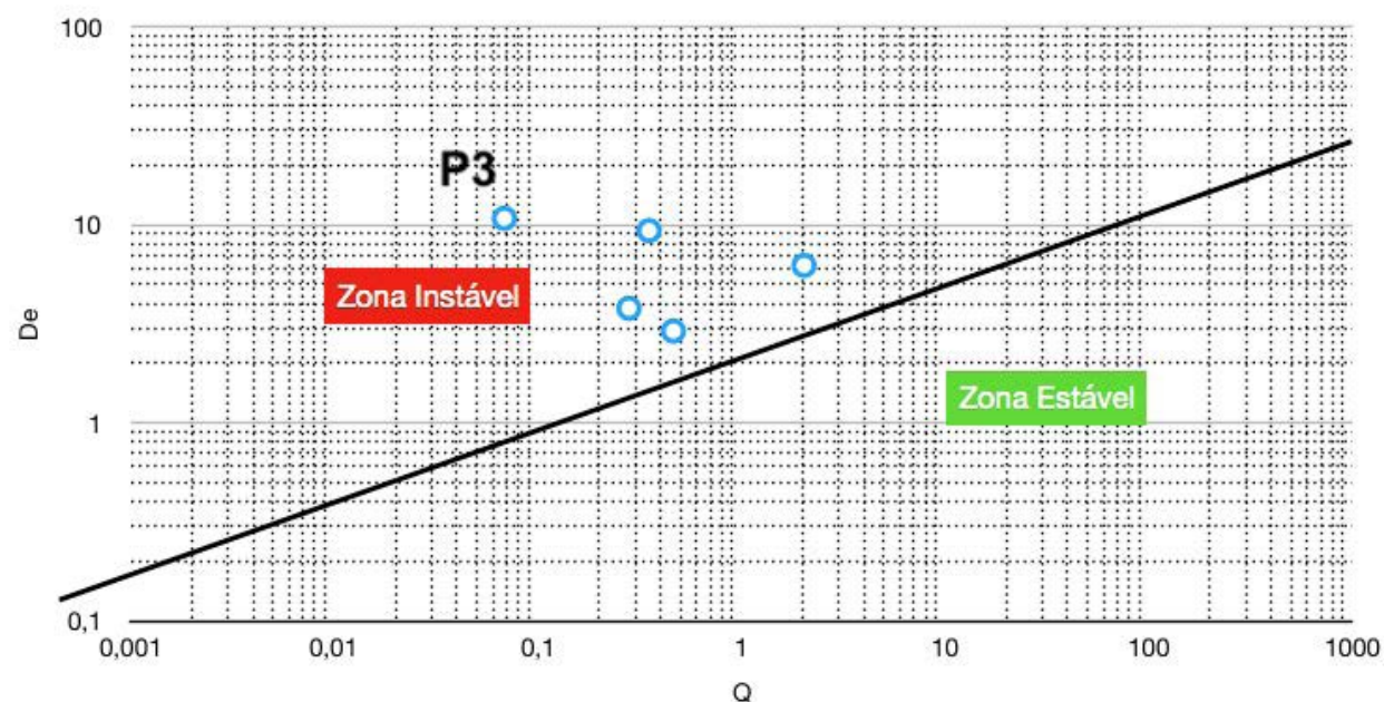
Figura 8: Gráfico de estabilidade geotécnica para os pontos amostrados. Em destaque os valores encontrados no P3, de menor valor do índice Q e maior diâmetro equivalente (De).
