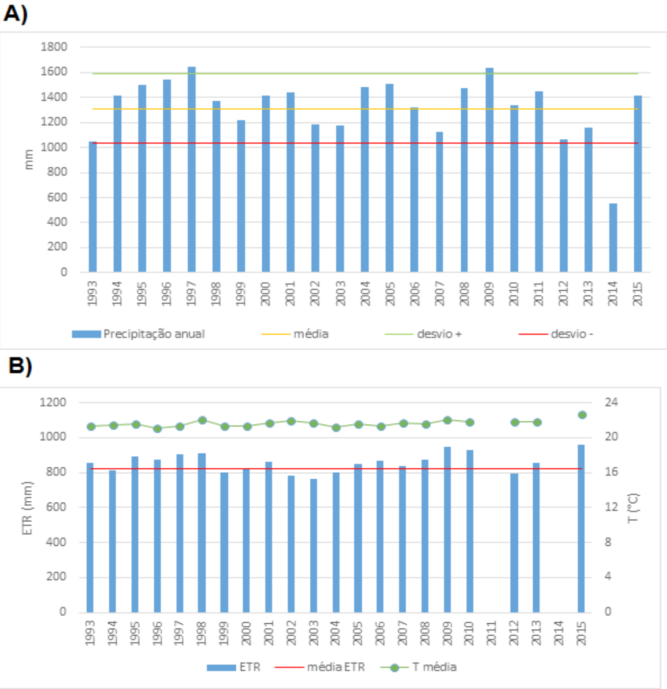
Figura 4 – Gráficos confeccionados a partir do balanço hídrico. A) Precipitação anual em milímetros durante o período 1993 - 2015, com a média e desvio padrão B) Evapotranspiração real anual em milímetros durante o período 1993 - 2015, e com a média e a variação da temperatura (°C).
