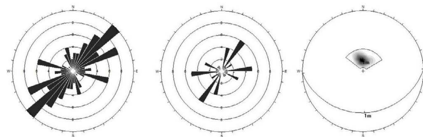
Figura 4: A: Roseta de direções de desenvolvimento dos condutos; B: Roseta de direções das fraturas observadas na cavidade; C: Estereograma de densidade de polos dos planos de acamamento medidos.
